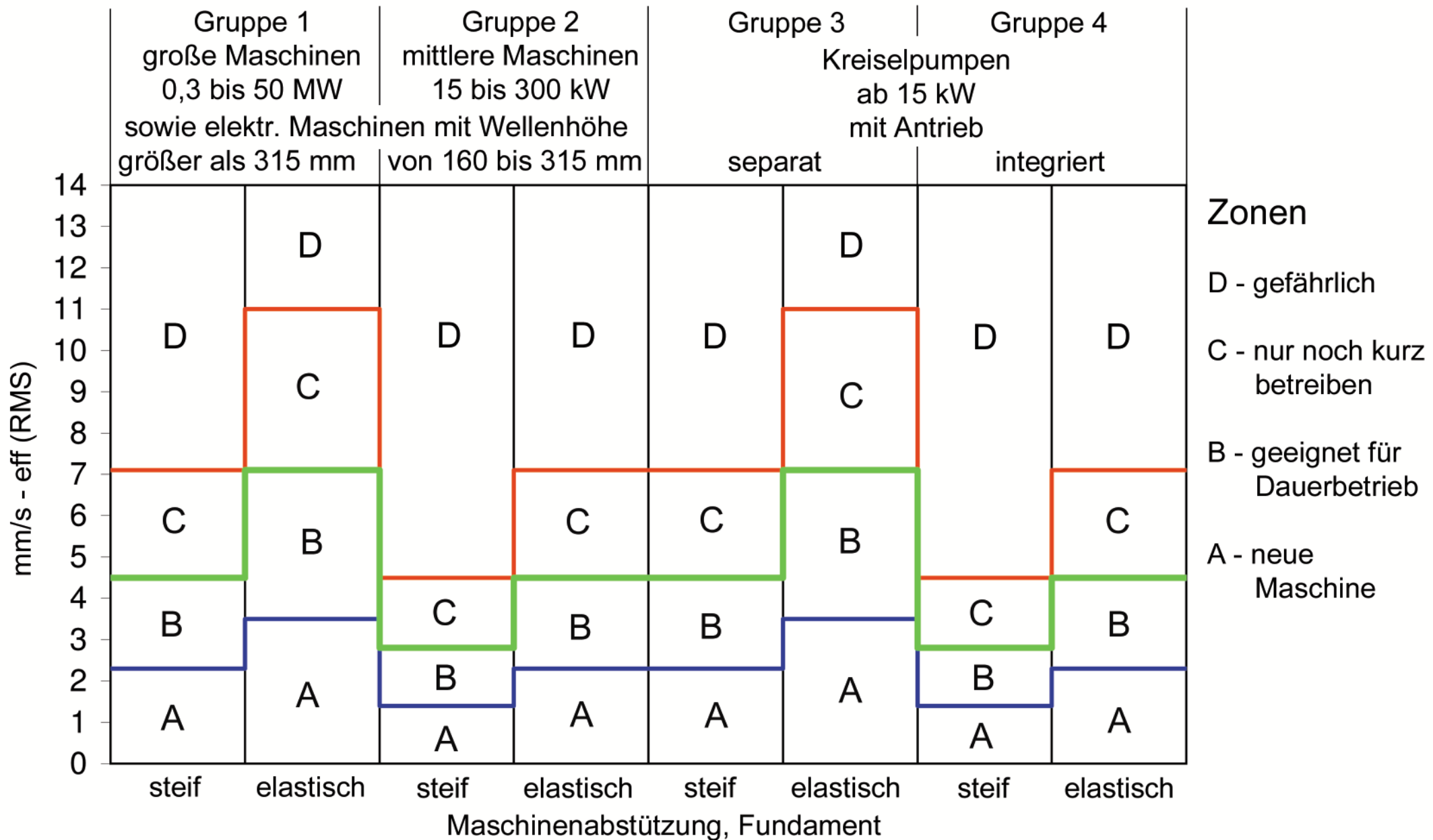
Bewertungszonen für Schwingstärken in mm/s - eff gemessen an Maschinen am Aufstellungsort (nach ISO 10816 - 3)
