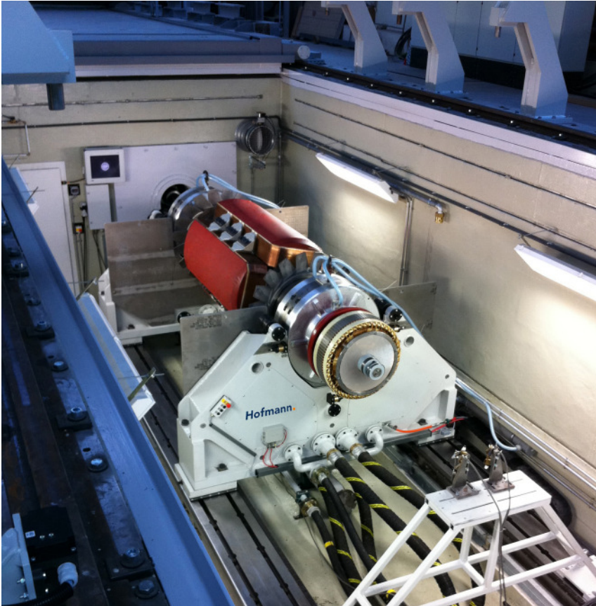
HS 28 für Turbogeneratoren, ausgeführt als Grube mit verfahrbarem Deckel.
